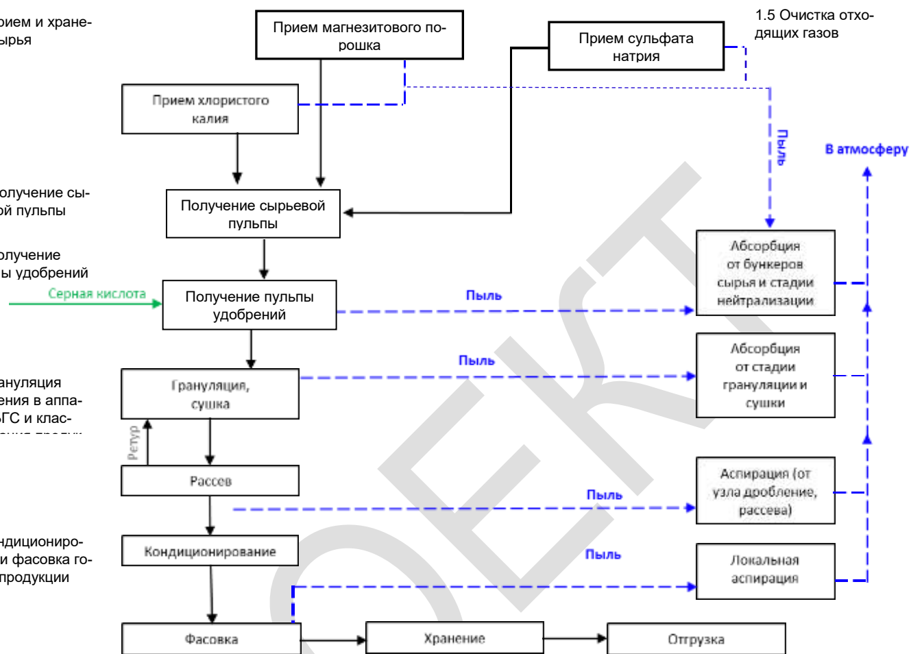
Рис. 6.1.9. Производство калийно-магниевого удобрения (калимаг)
