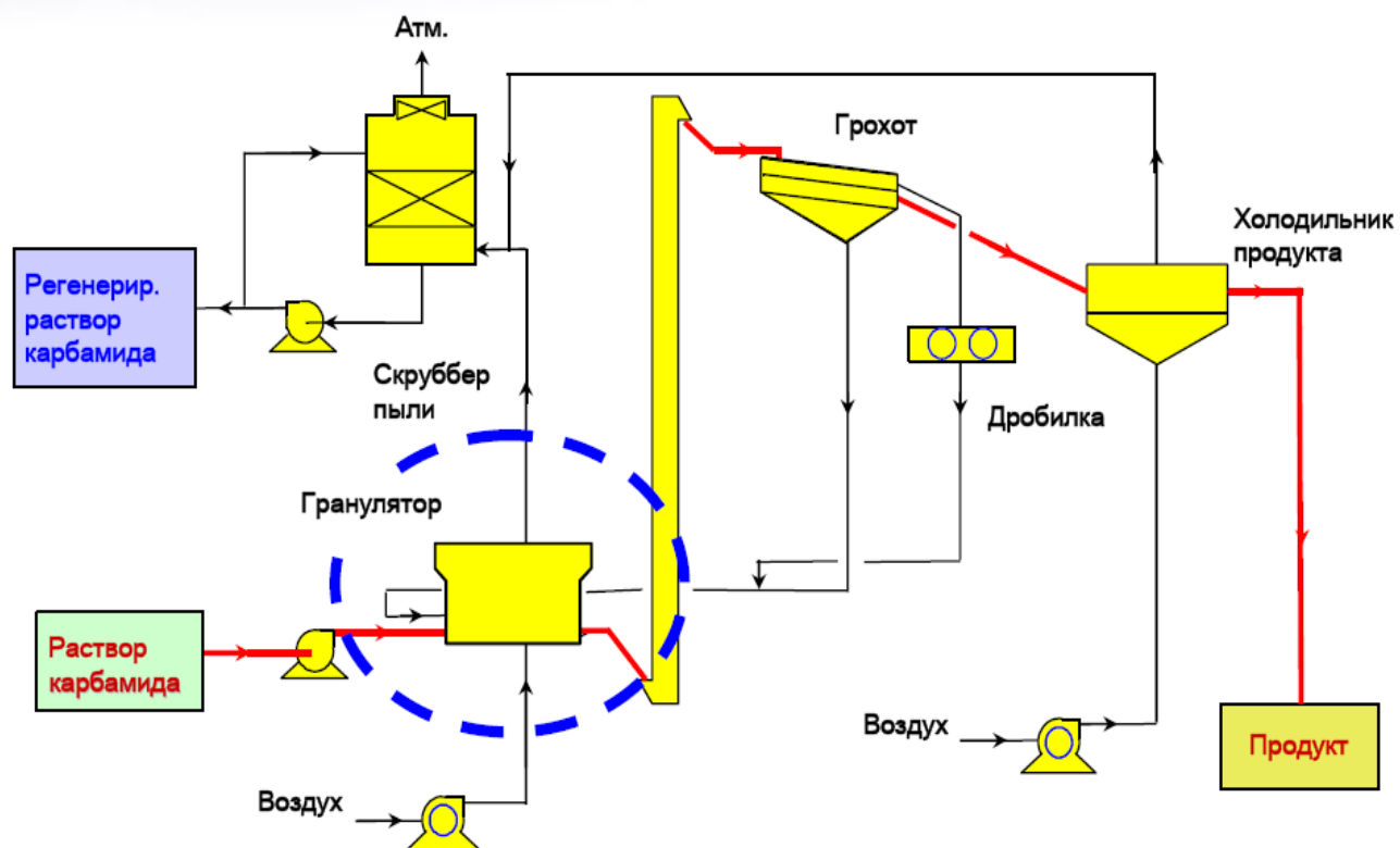
Рисунок 8.20 — Принципиальная технологическая схема процесса грануляции ТЕС
