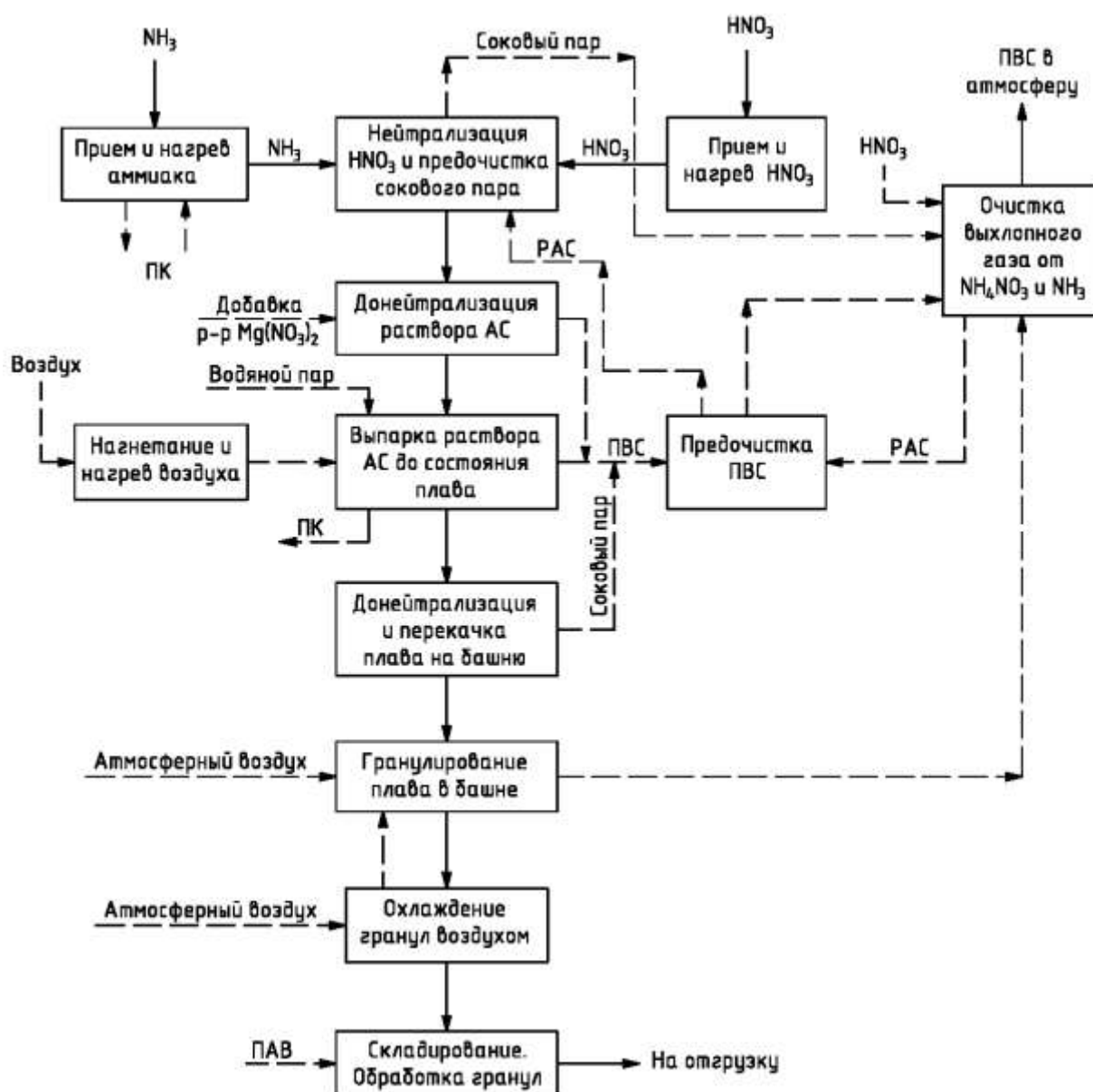
Рисунок 7.2 — Описание схемы технологического процесса в агрегатах АС-72М
