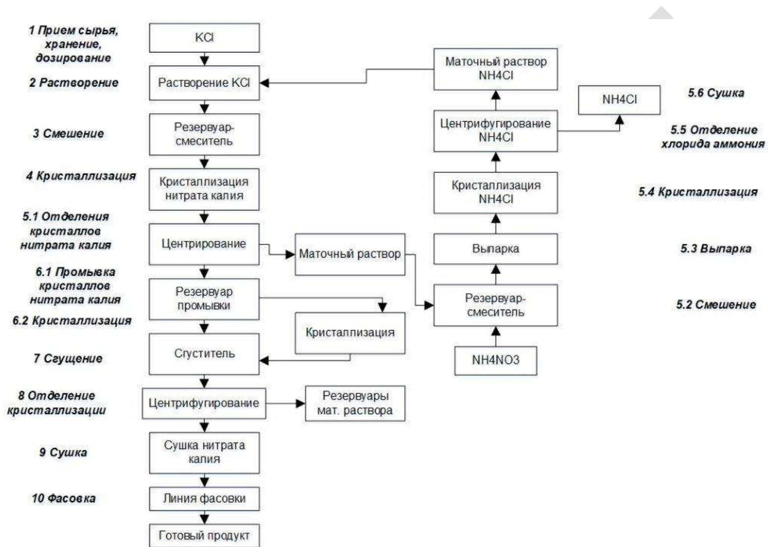
Рис. Схема производства нитрата калия из хлорида калия и нитрата аммония
