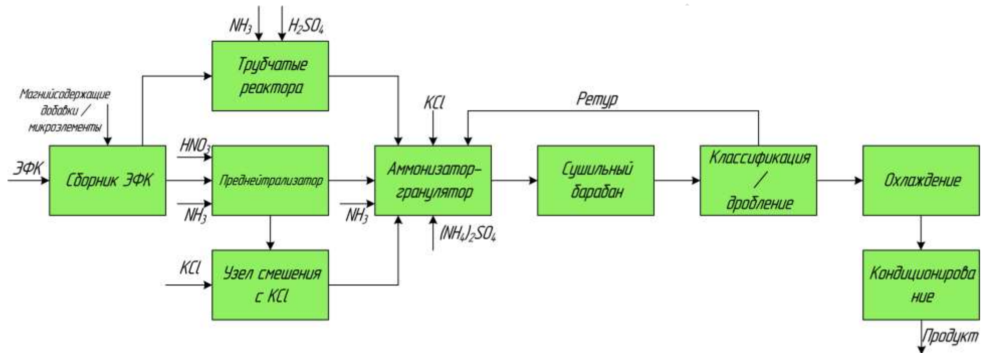
Рис. Технология гранулированных нитратсодержащих NPK-удобрений на основе нейтрализации смеси азотной и фосфорной кислот с последующим гранулированием и сушкой по схеме АГ-СБ
