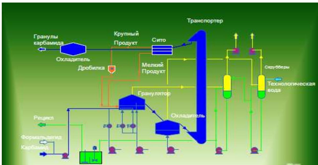
Рисунок 8.36 — Принципиальная схема гранулирования карбамида по технологии Stamicarbon
