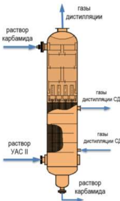
Рисунок 8.5 — Дистиллятор низкого давления
