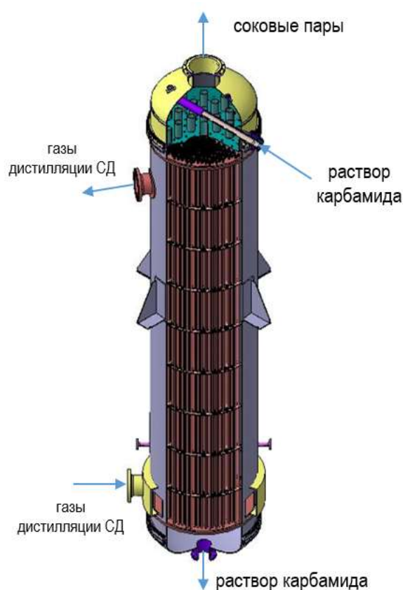
Рисунок 8.6 — Теплообменник-рекуператор
