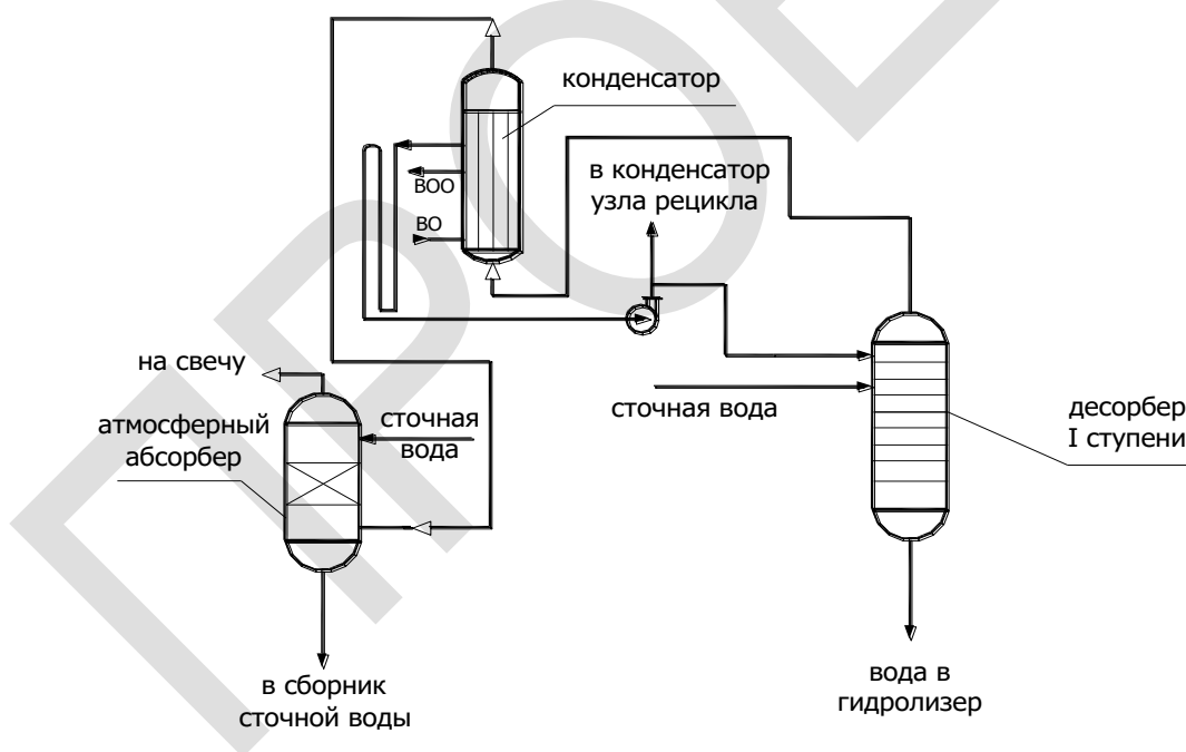
Рисунок 8.33 — Схема установки затопленного конденсатора газов десорбции
