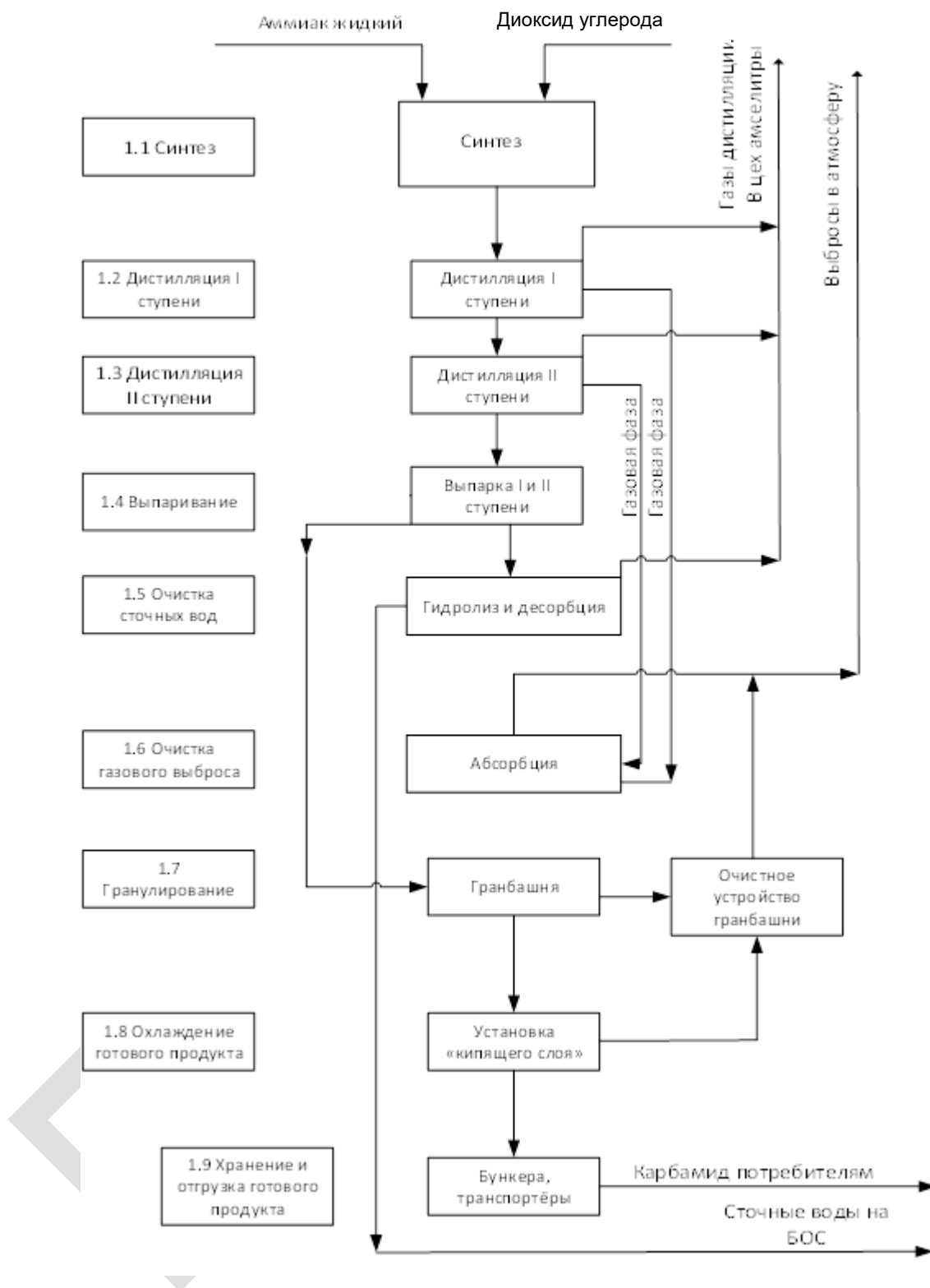
Рисунок 8.2 — Схема технологического процесса (включая получение готового продукта).
