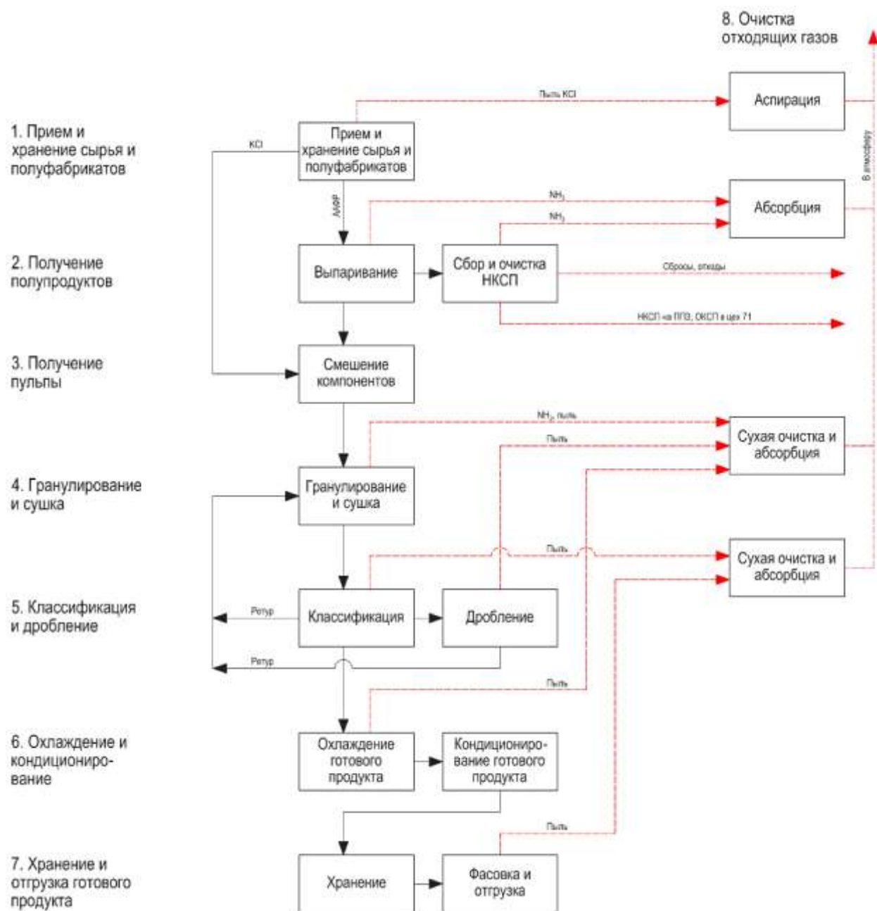
Рисунок 6.8 — Получение NPK-удобрений
