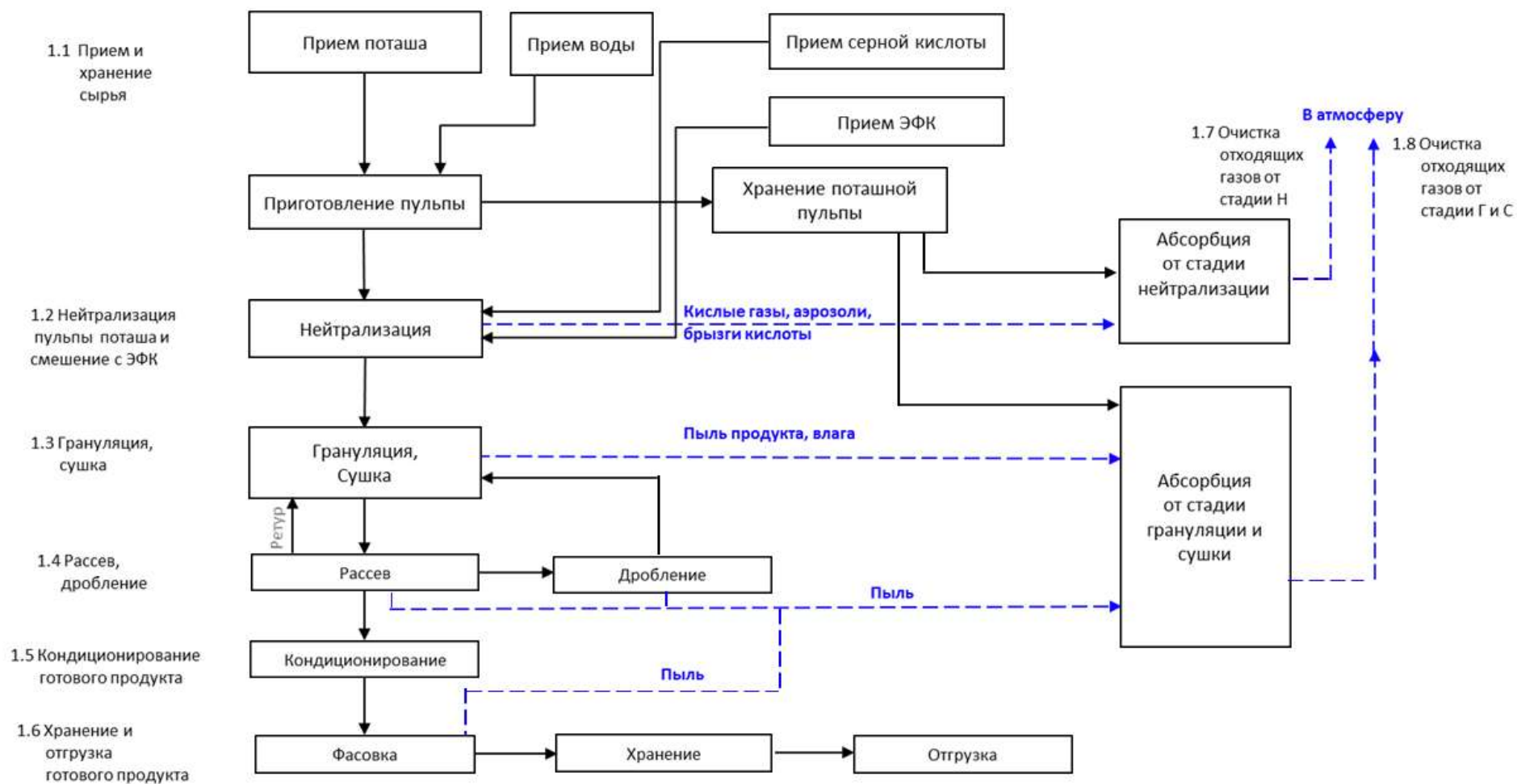
Рисунок 6.15 — Производство сульфата калия
