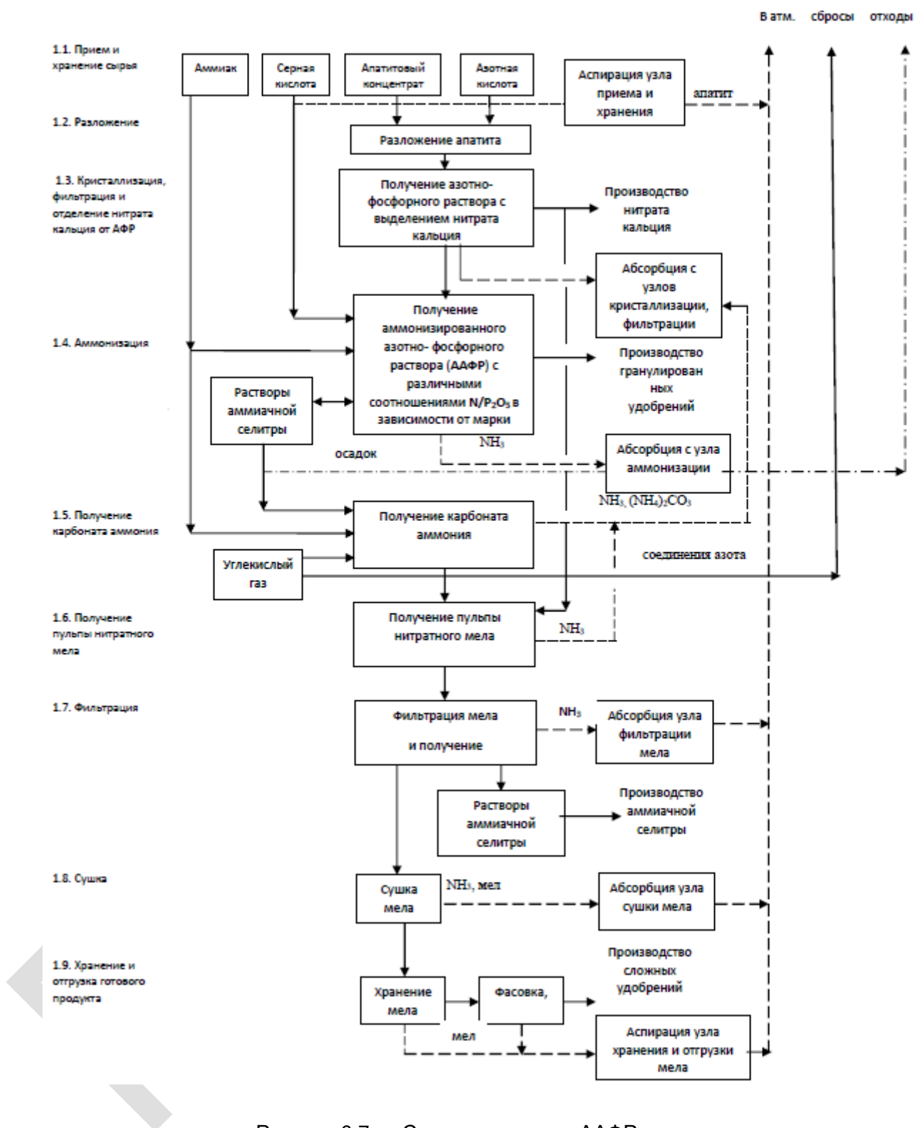
Рисунок 6.7 — Схема получения ААФР
