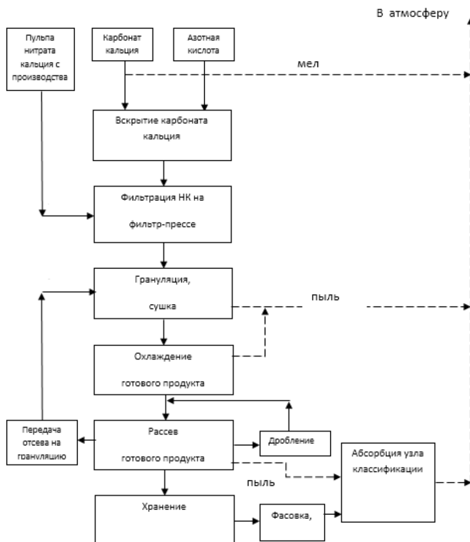
Рисунок 6.11 — Процесс производства нитрата кальция
