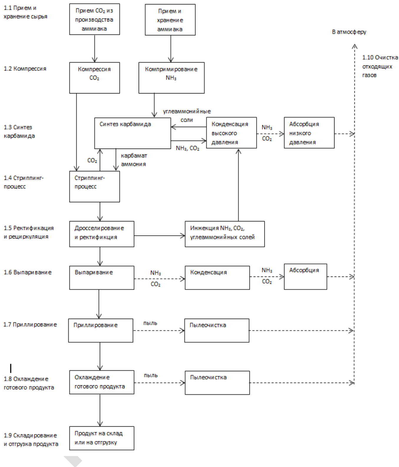
Рисунок 8.7 — Схема технологического процесса (включая получение готового продукта)
