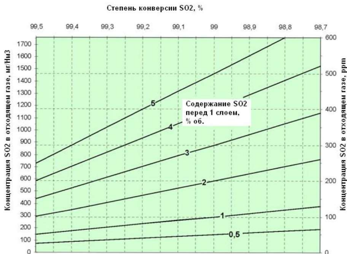
Рисунок 3.3 — Зависимость концентрации \text{SO}_2 в отходящих газах сернокислотных установок от степени контактирования при начальном содержании \text{SO}_2 в технологическом газе 0,5–5 об. %.
