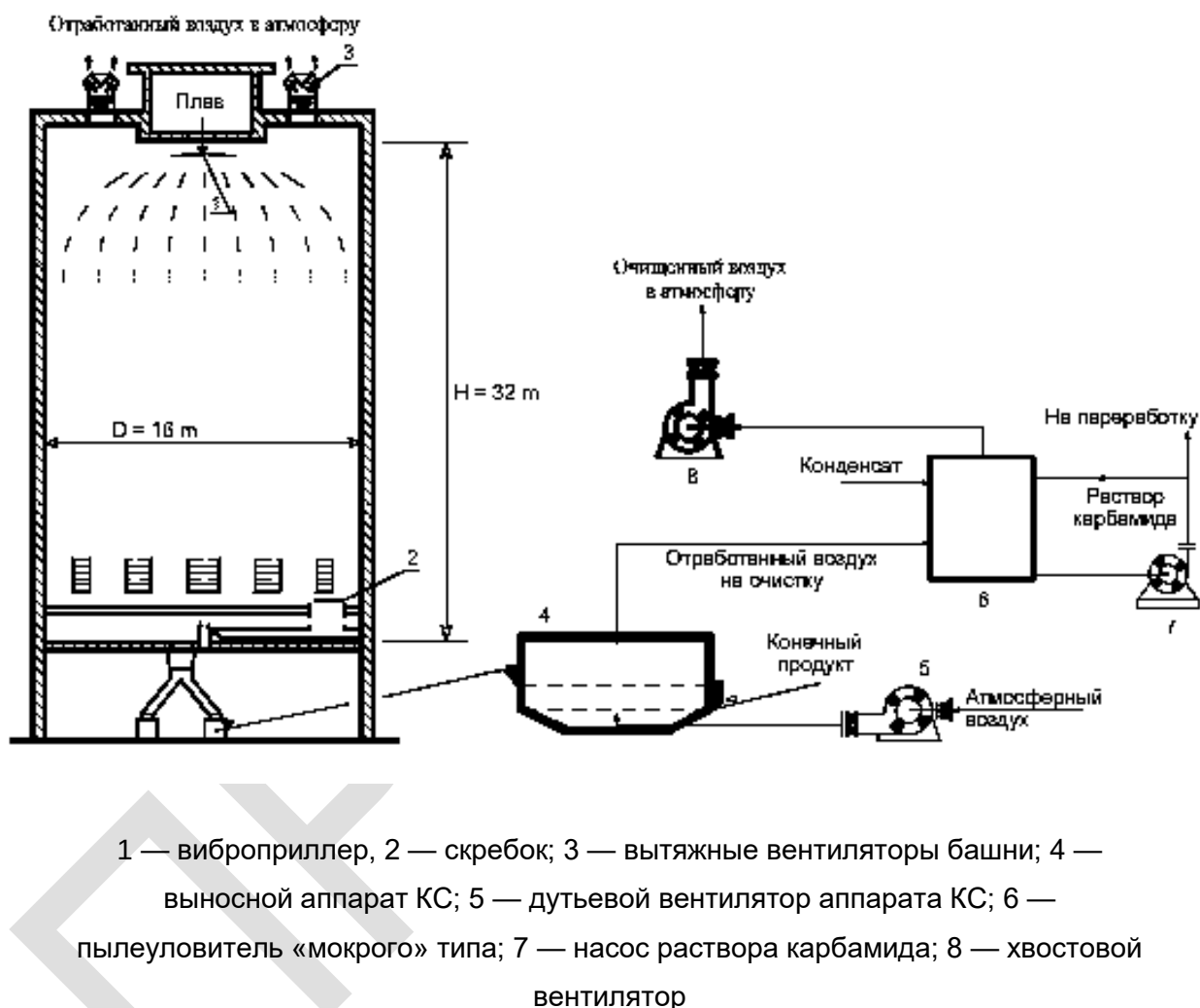
Рисунок 8.11 — Принципиальная схема узла прилливания после реализации мероприятий по модернизации башен
