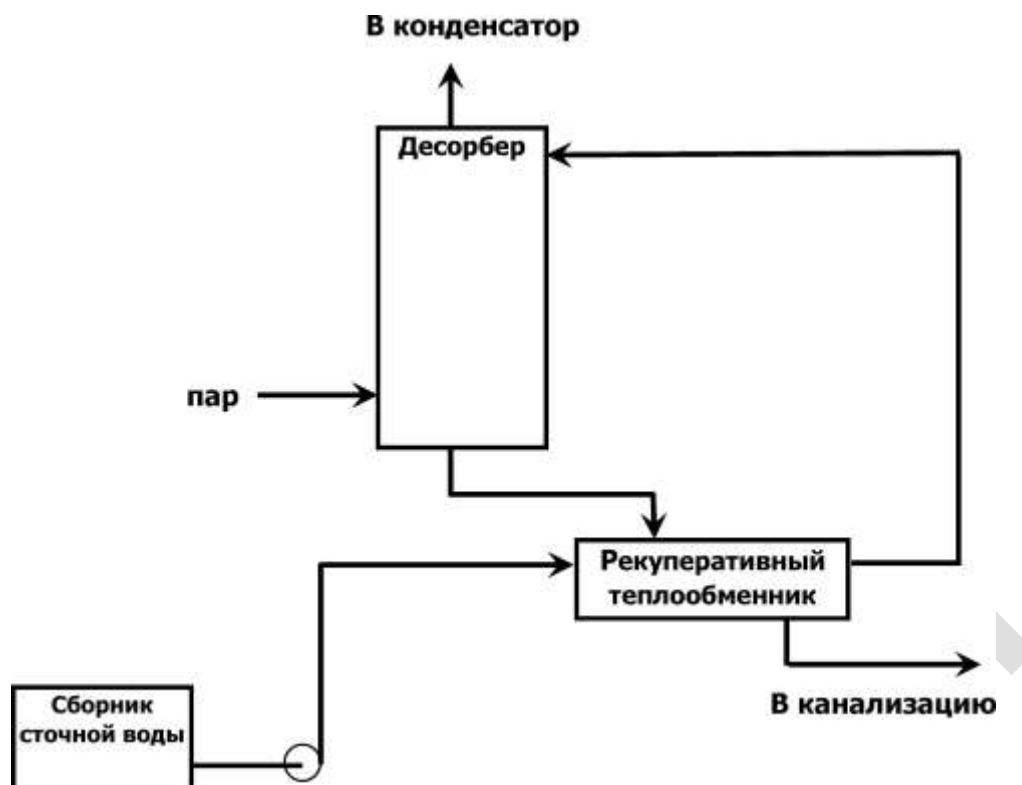
Рисунок 8.25 — Принципиальная схема десорбции аммиака в одну ступень
