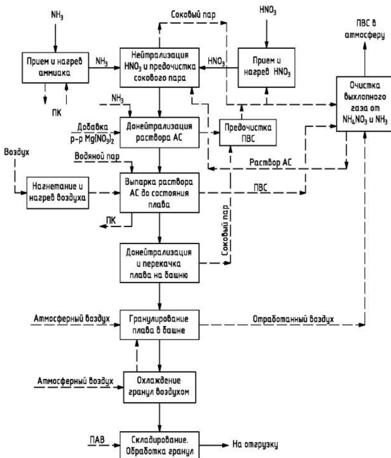
Рисунок 7.1 — Описание схемы технологического процесса в агрегатах АС-72
