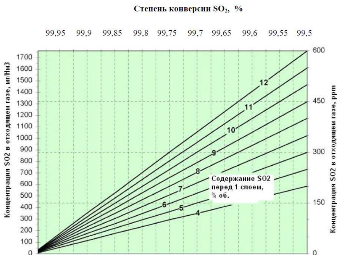
Рисунок 3.2 — Зависимость концентрации \text{SO}_2 в отходящих газах сернокислотных установок от степени контактирования при начальном содержании \text{SO}_2 в технологическом газе 4–12 об. %.
