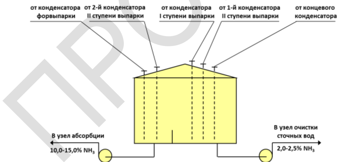
Рисунок 8.34 — Пример перераспределения потоков процессного конденсата (КСП)
