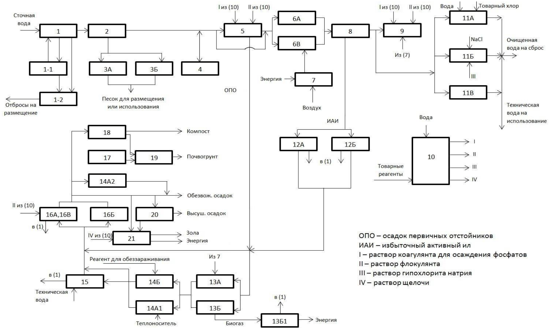
Рисунок 2.2 — Обобщенная технологическая схема
