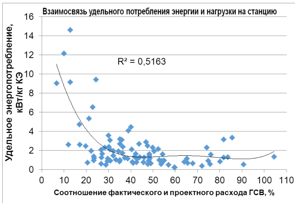
Рисунок 0.1 — Зависимость удельного энергопотребления от нагрузки на ОС ГСВ по сточным водам
