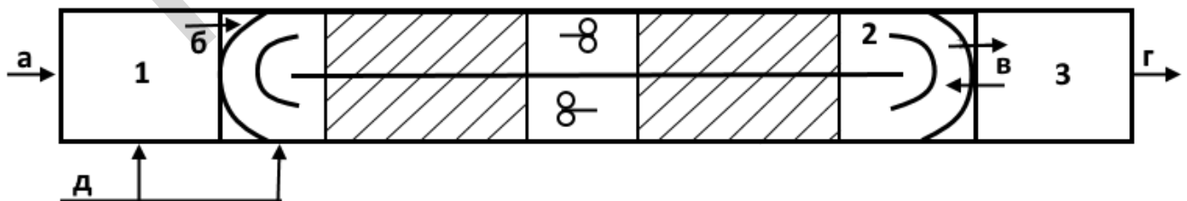
«Карусельная нитри–денитрификация». На примере демонстрационной линии на Курьяновских ОС (Москва), 1995–1998 годы, 40 тыс. м 3 /сут
