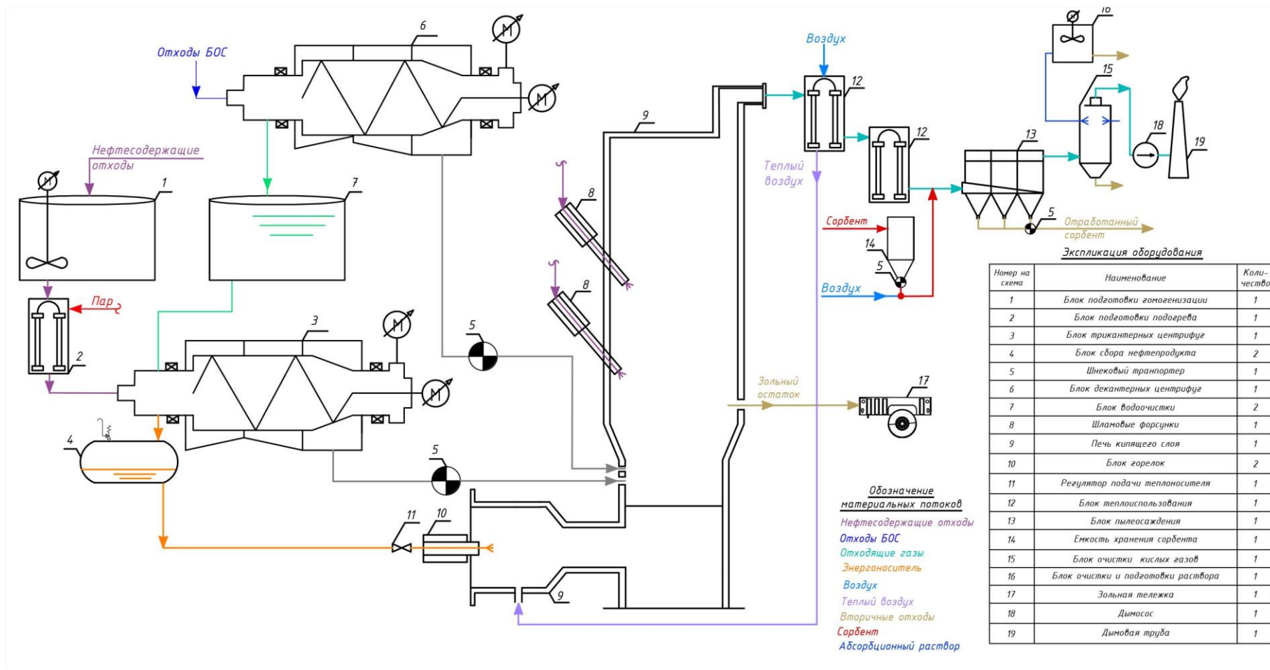
Рисунок 2.26 — Технологическая схема комбинации физико-химической обработки отходов и сжигания
