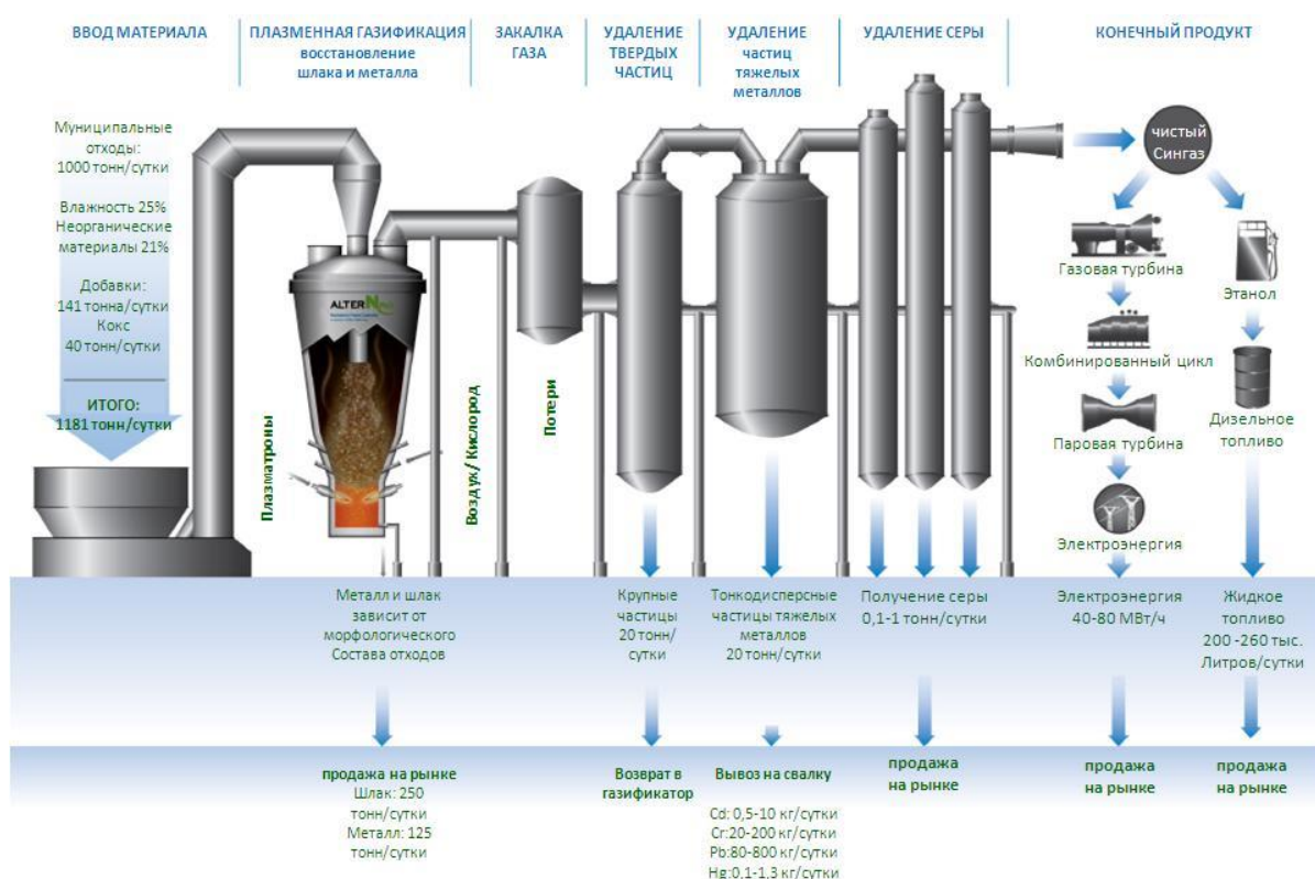
Рисунок 2.34 – Технологическая схема плазменной газификации
