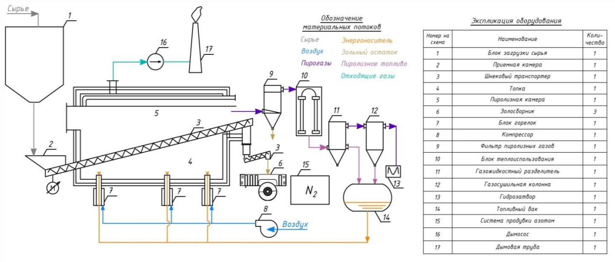
Рисунок 2.18 — Технологическая схема пиролиза с получением печного топлива
