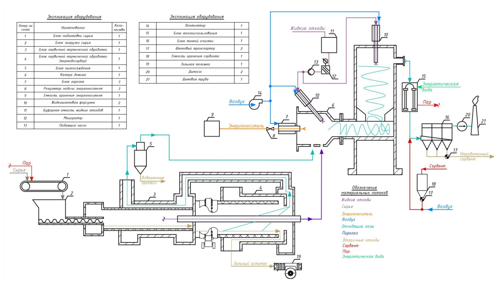
Рисунок 2.25 — Технологическая схема комбинации пиролиза, термодесорбции, сжигания
