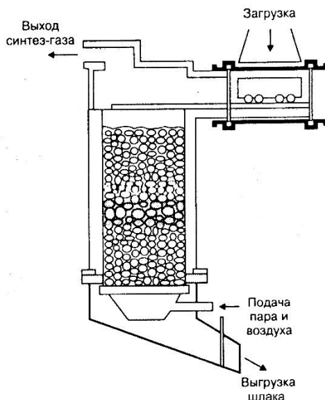
Рисунок 2.10 — Шахтная печь [19]
