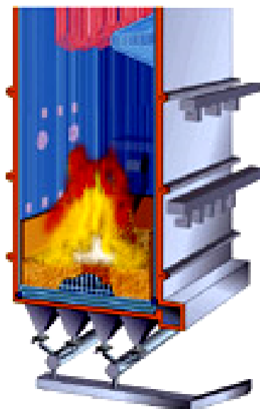
Рисунок 2.14 — Топка с кипящим слоем [11]
