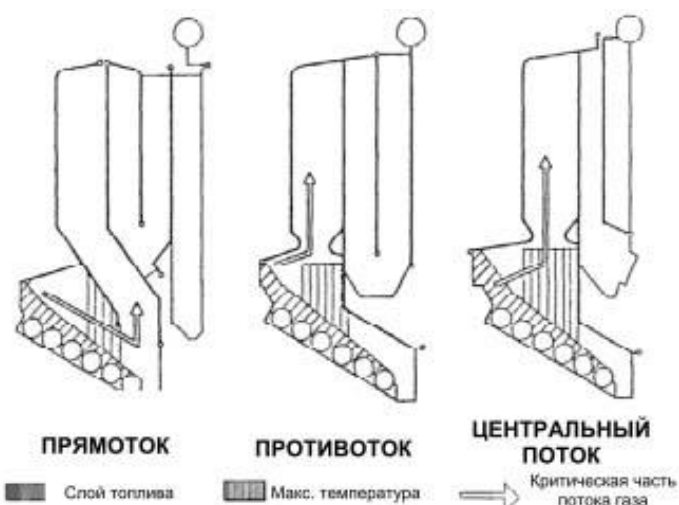
Рисунок 2.5 – Варианты проводки дымовых газов [62]
