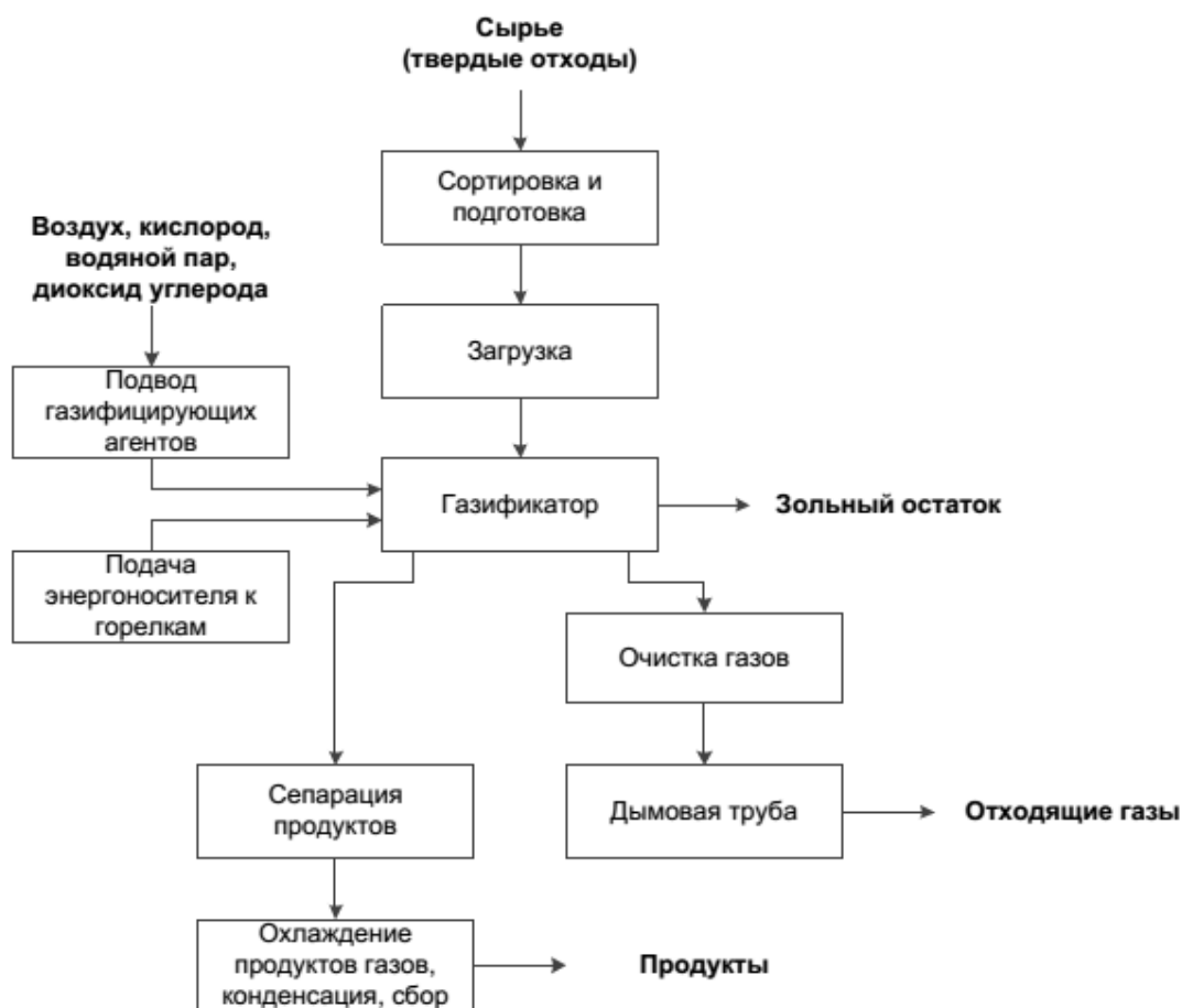
Рисунок 2.22 – Общая схема газификации отходов
