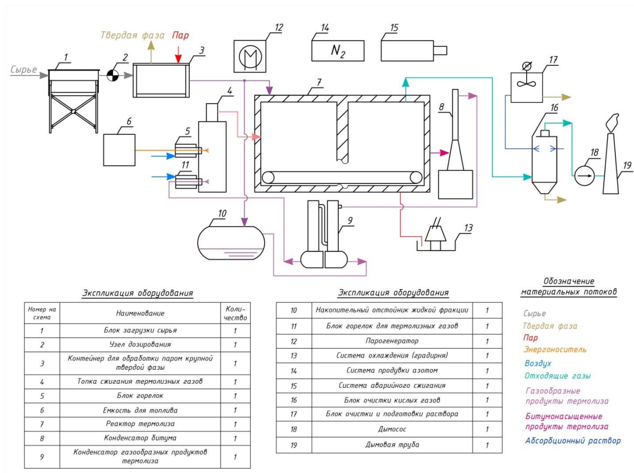
Рисунок 2.20 — Технологическая схема термоллизной переработки нефтешламов
