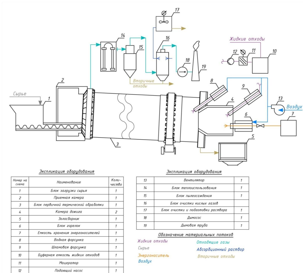
Рисунок 2.8 — Принципиальная технологическая схема сжигания отходов с использованием циклонного дожигателя
