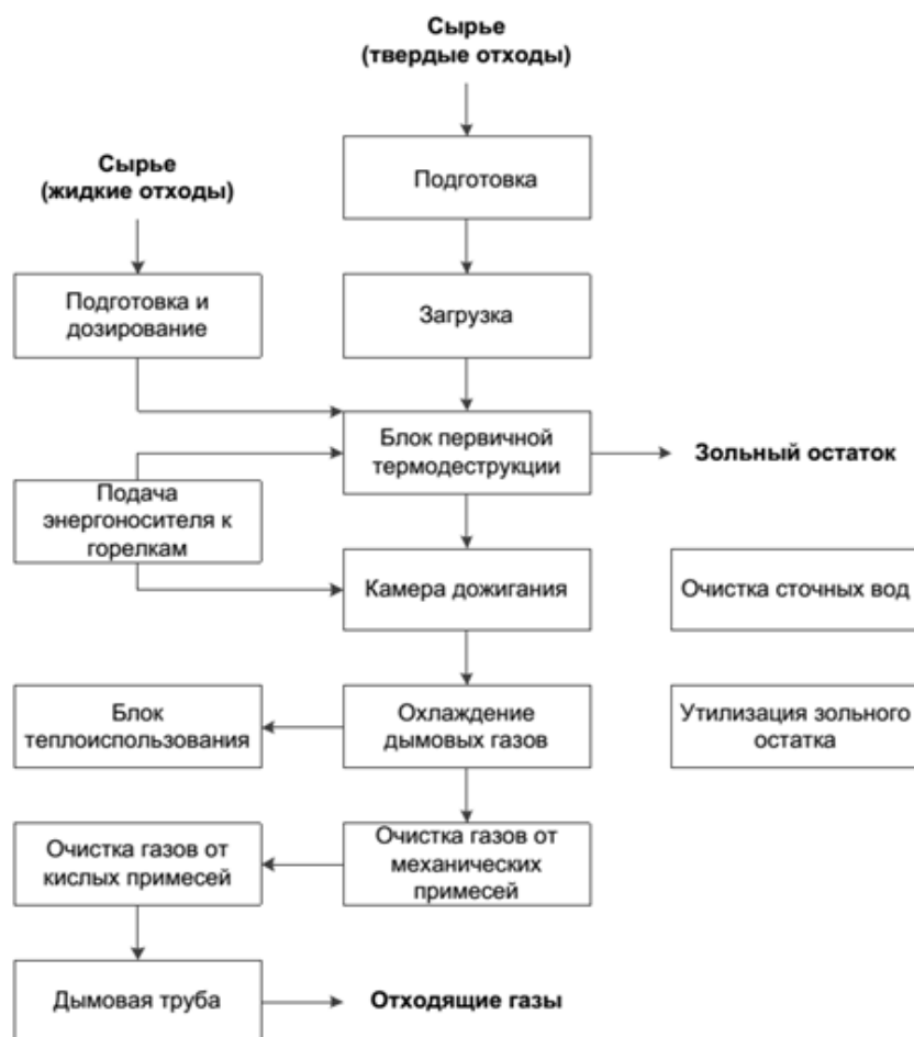
Рисунок 2.1 – Общая схема сжигания отходов с целью обезвреживания
