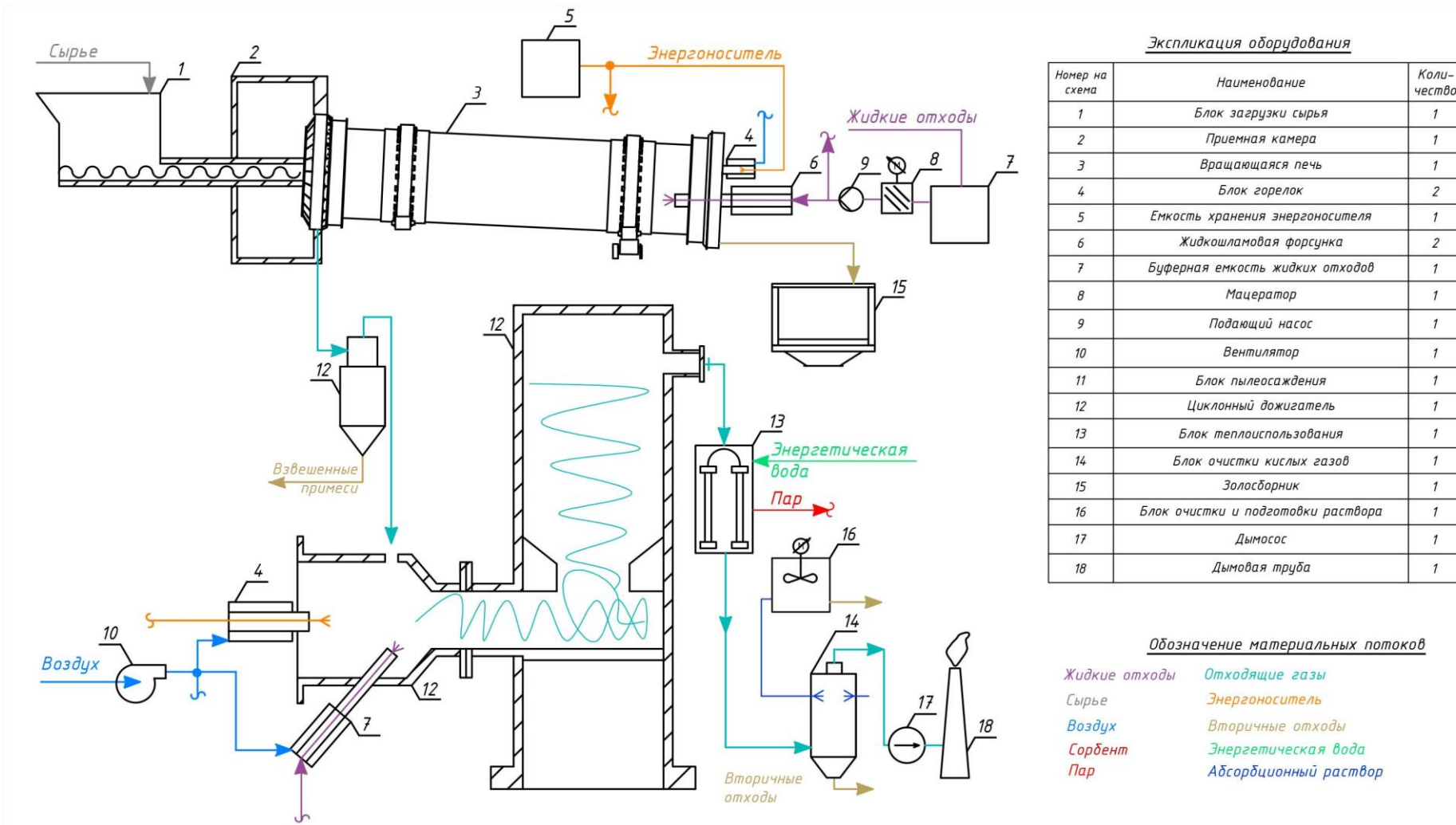
Рисунок 2.21 — Технологическая схема высокотемпературного пиролиза
