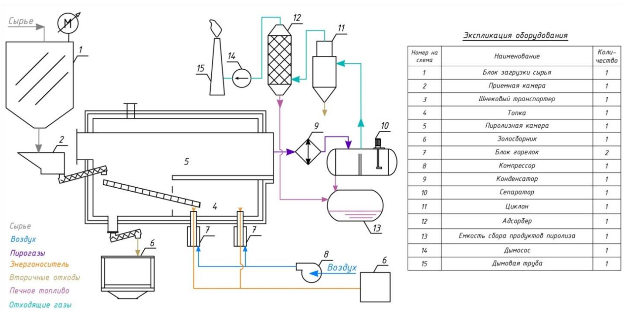
Рисунок 2.19 — Технологическая схема пиролиза с получением топлива
