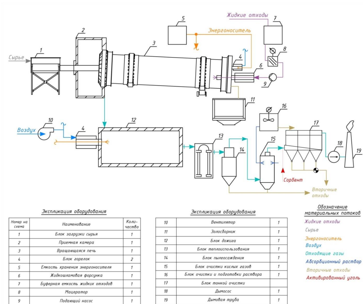
Рисунок 2.7 — Принципиальная технологическая схема сжигания отходов во вращающейся барабанной печи)
